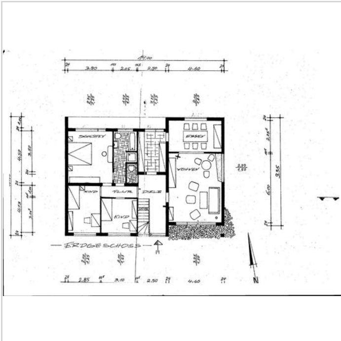
Grundriss EG
