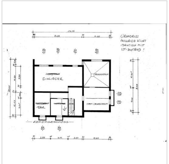
Grundriss KG
